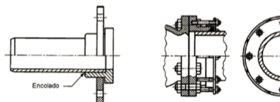
Figura 29 - União por flange
