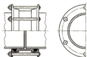
Figura 28 - União mecânica
